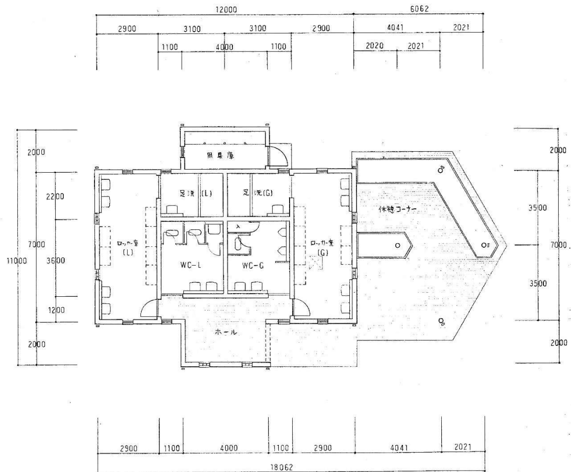
平面図
