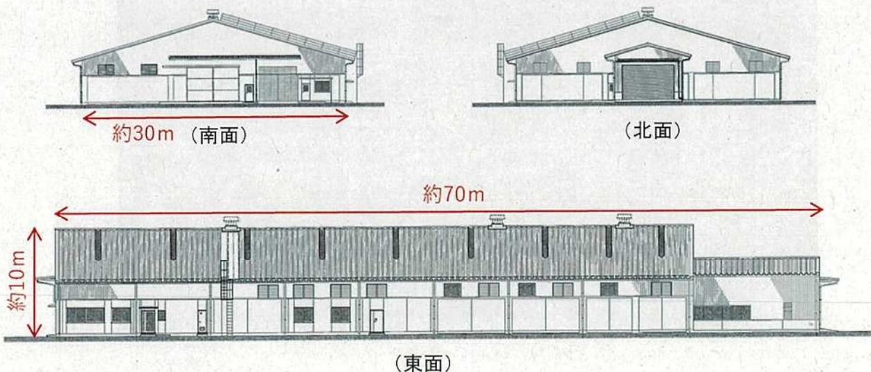
コンポスト化施設 立面図
