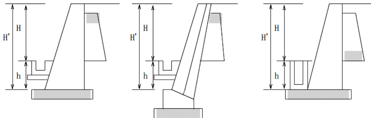
図 10-24 排水構造物がある場合の根入れ
