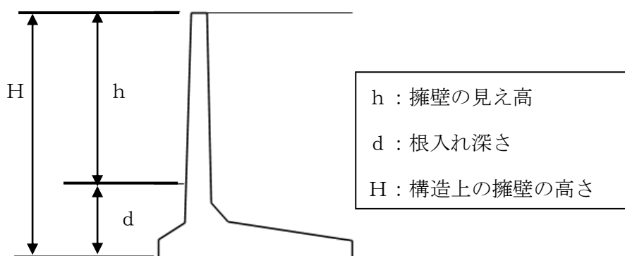
図 10-23 擁壁の根入れ
