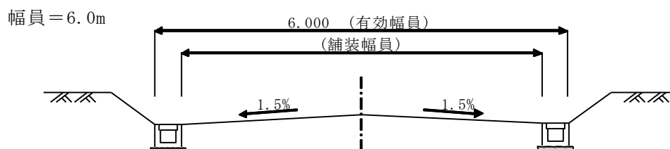
図3-2 有効幅員のとらえ方
