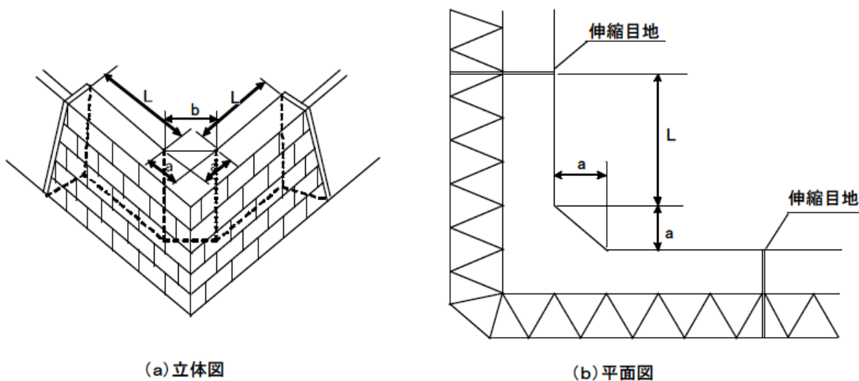
図 10-16 隅角部の補強方法および伸縮継目の位置
