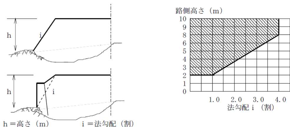
図 3-13 法勾配と路側高さの関係
