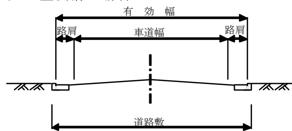
図 3 - 3 道路各部の名称
