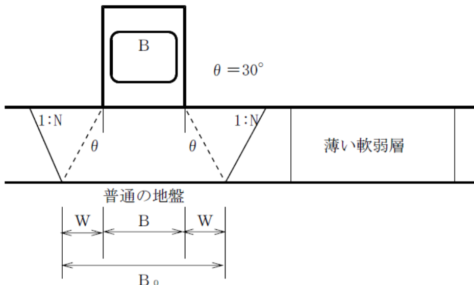
図 3-12 置換基礎
