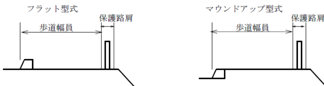
図 3-10 歩道の形式
