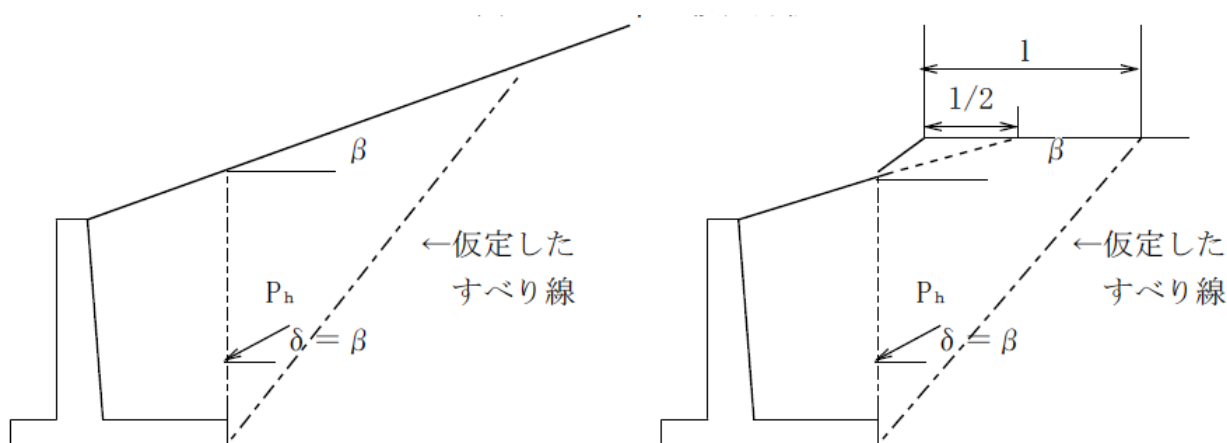
図 10-11 \beta の設定方法
