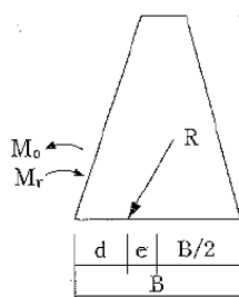
(a) 重力式擁壁の場合
