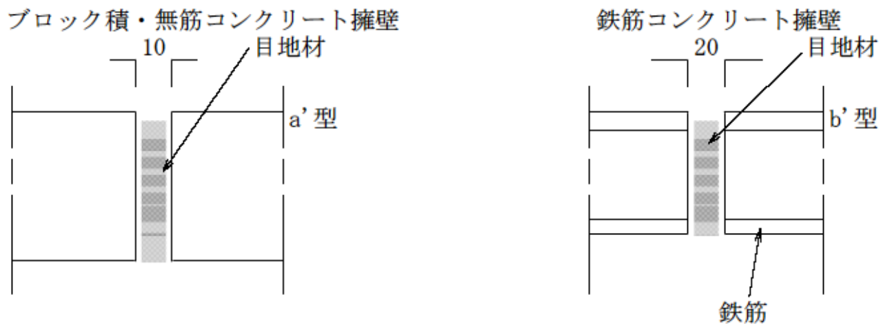
図 10-25 伸縮目地
