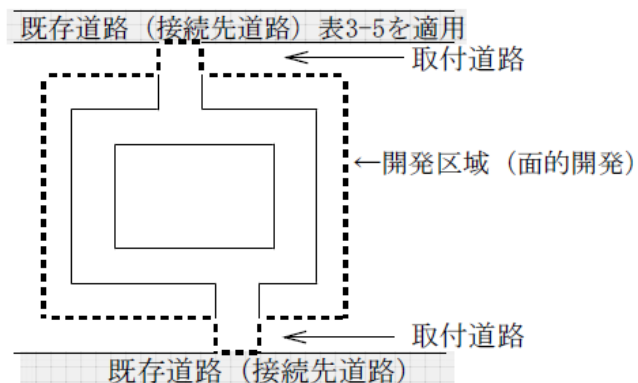
図 3-5 接続道路
