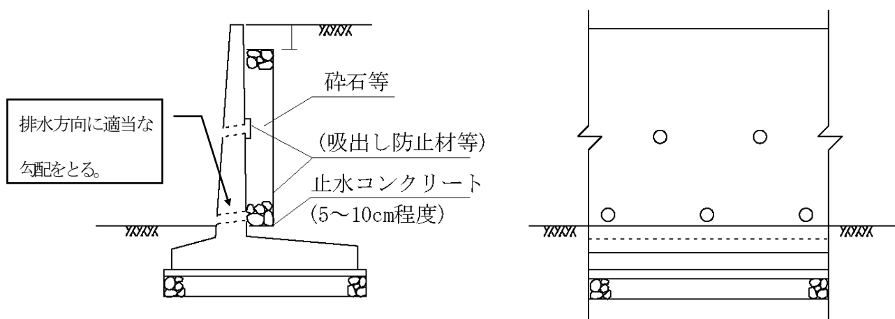
図 10-22 水抜き穴の設置
