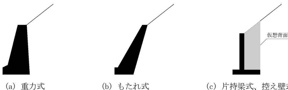
図 10-10 擁壁の自重
