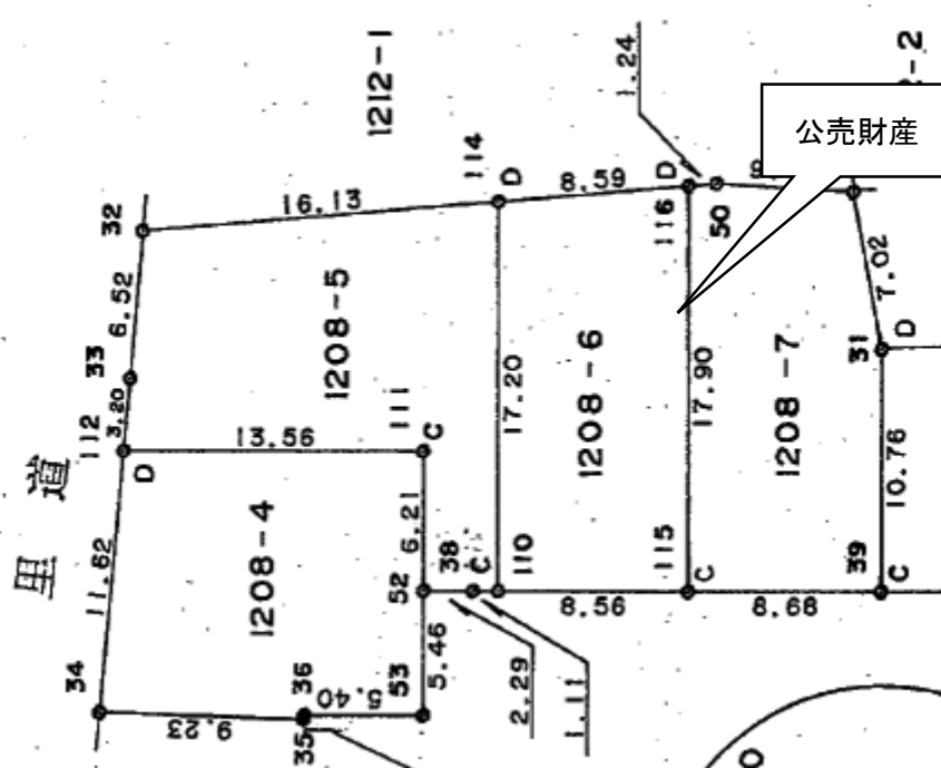
地積測量図
