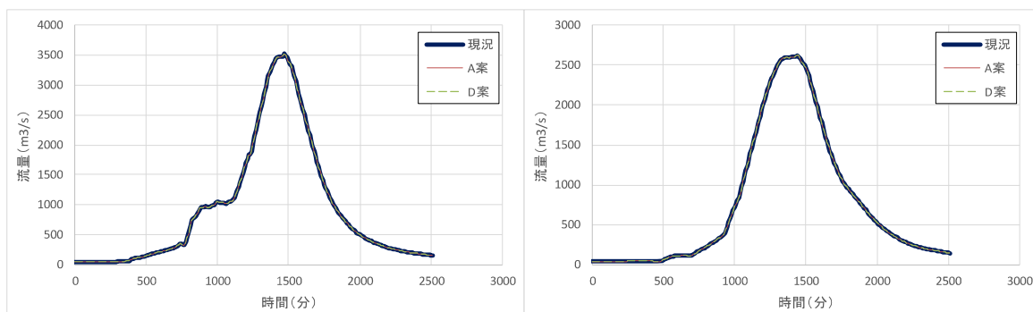
図 1-1-20 北川合流後地点の時系列流量グラフ（左：200 年確率、右：H25.9）
