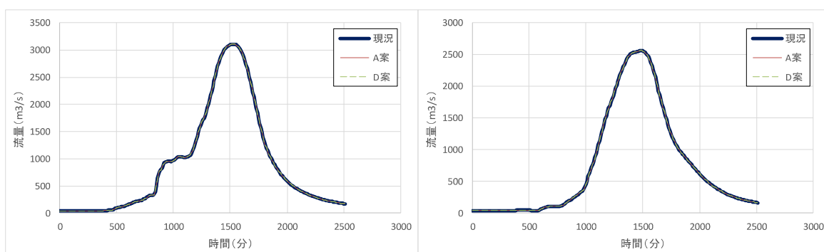
図 1-1-17 常安橋地点の時系列流量グラフ（左：200 年確率、右：H25.9）
