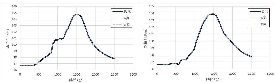
図 1-1-13 常安橋地点の時系列水位グラフ（左：200 年確率、右：H25.9）
