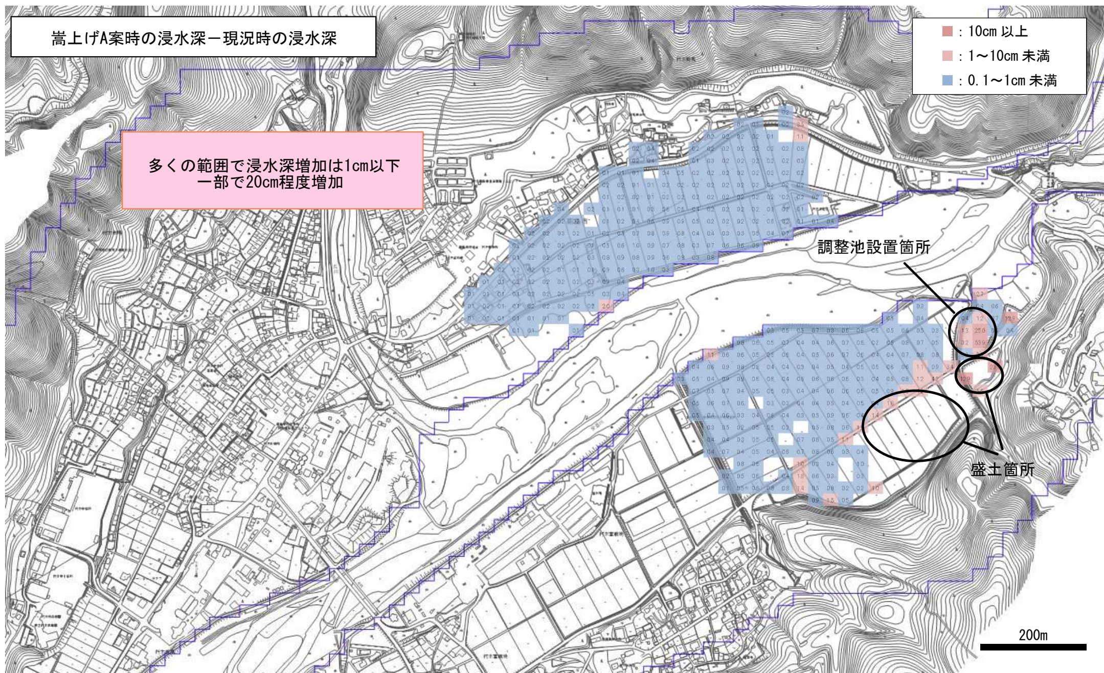
嵩上げA案時と現況時の浸水深差分図（200年確率流量）
