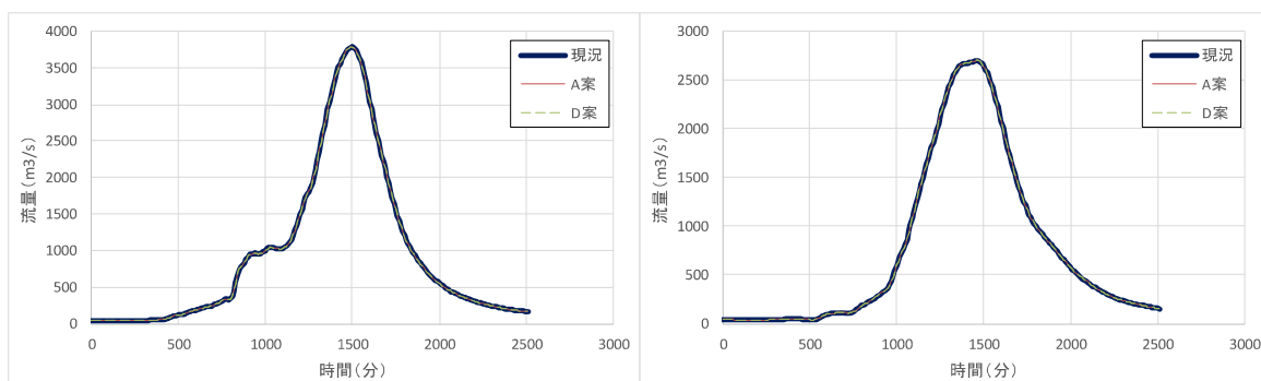
図 1-1-18 両台橋地点の時系列流量グラフ（左：200 年確率、右：H25.9）
