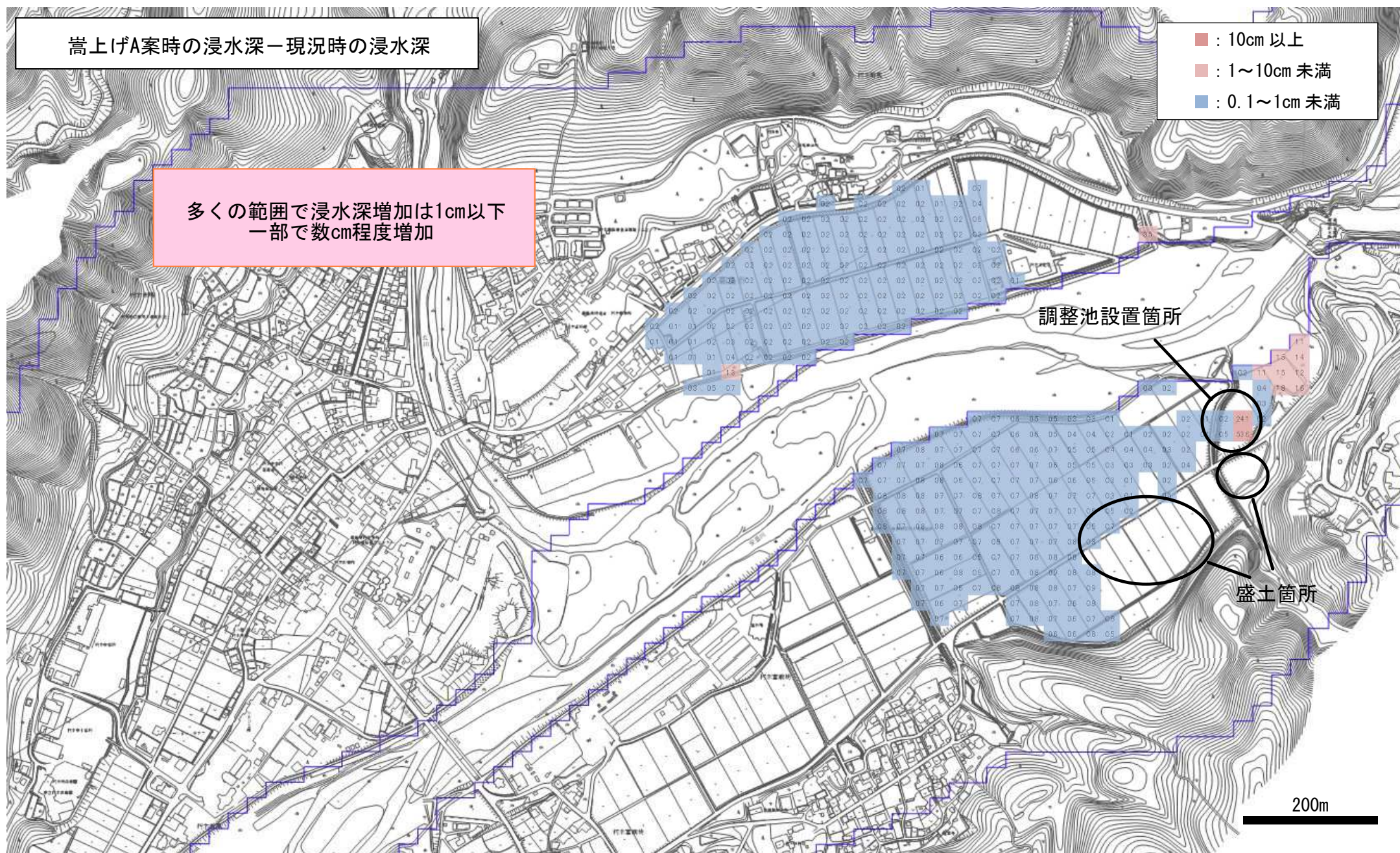
嵩上げA案時と現況時の浸水深差分図（平成25年9月流量）
