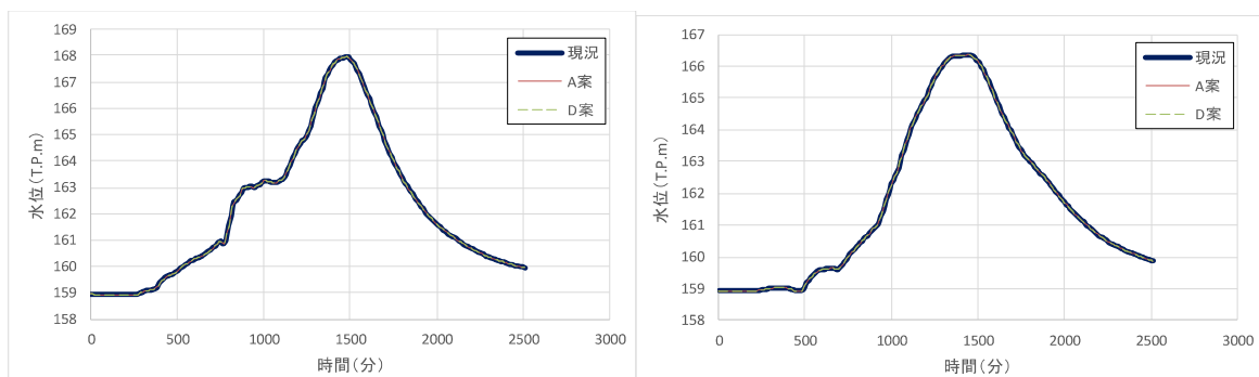
図 1-1-15 ごみ処理施設近傍の河道地点の時系列水位グラフ（左：200 年確率、右：H25.9）
