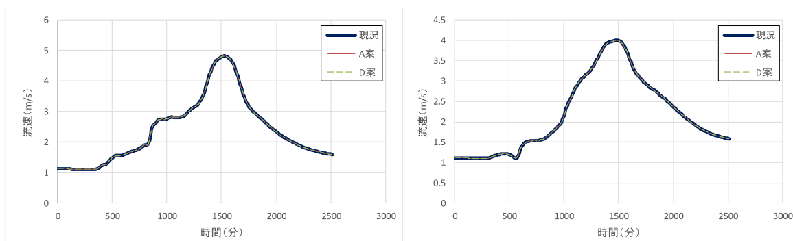
図 1-1-21 常安橋地点の時系列流速グラフ（左：200 年確率、右：H25.9）
