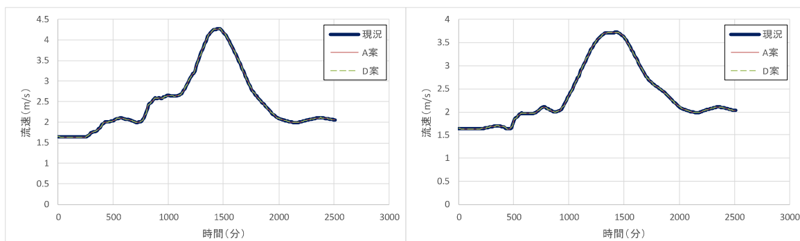
図 1-1-24 北川合流後地点の時系列流速グラフ（左：200 年確率、右：H25.9）
