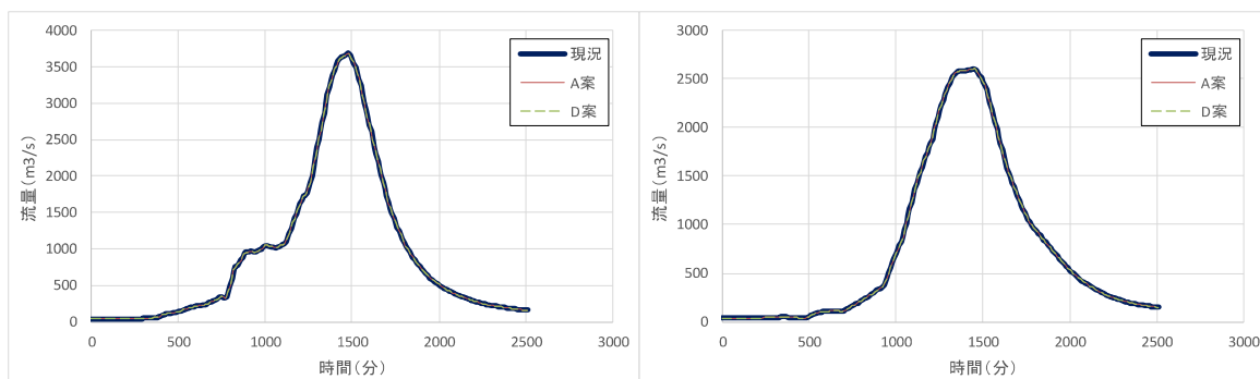
図 1-1-19 ごみ処理施設近傍の河道地点の時系列流量グラフ（左：200 年確率、右：H25.9）
