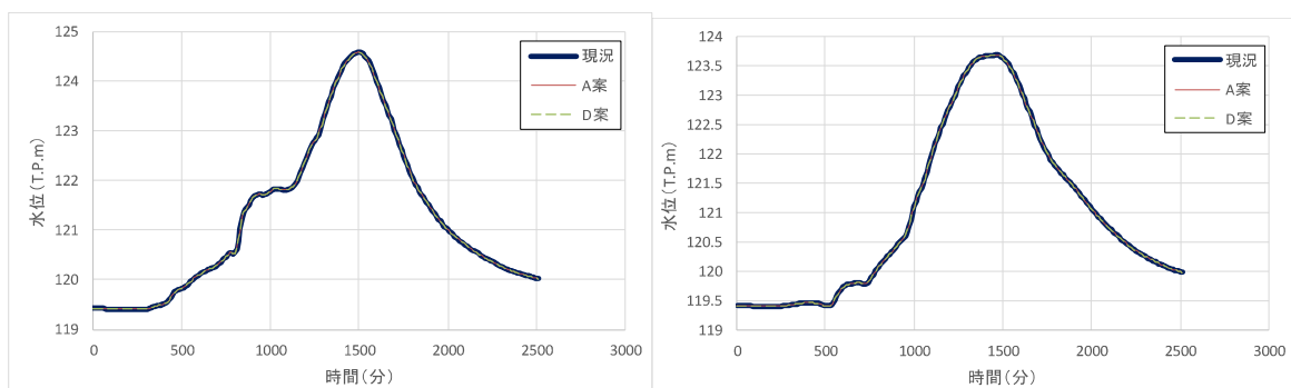
図 1-1-14 両台橋地点の時系列水位グラフ（左：200 年確率、右：H25.9）
