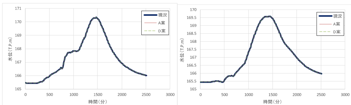
図 1-1-16 北川合流後地点の時系列水位グラフ（左：200 年確率、右：H25.9）
