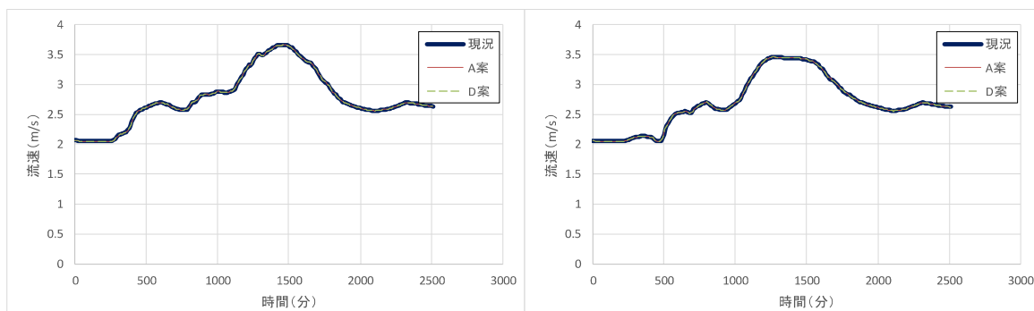
図 1-1-23 ごみ処理施設近傍の河道地点の時系列流速グラフ（左：200 年確率、右：H25.9）
