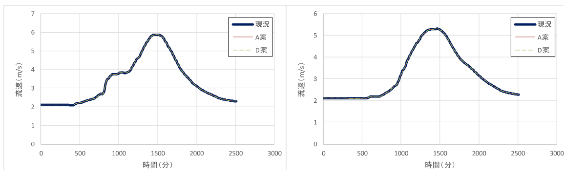
図 1-1-22 両台橋地点の時系列流速グラフ（左：200 年確率、右：H25.9）
