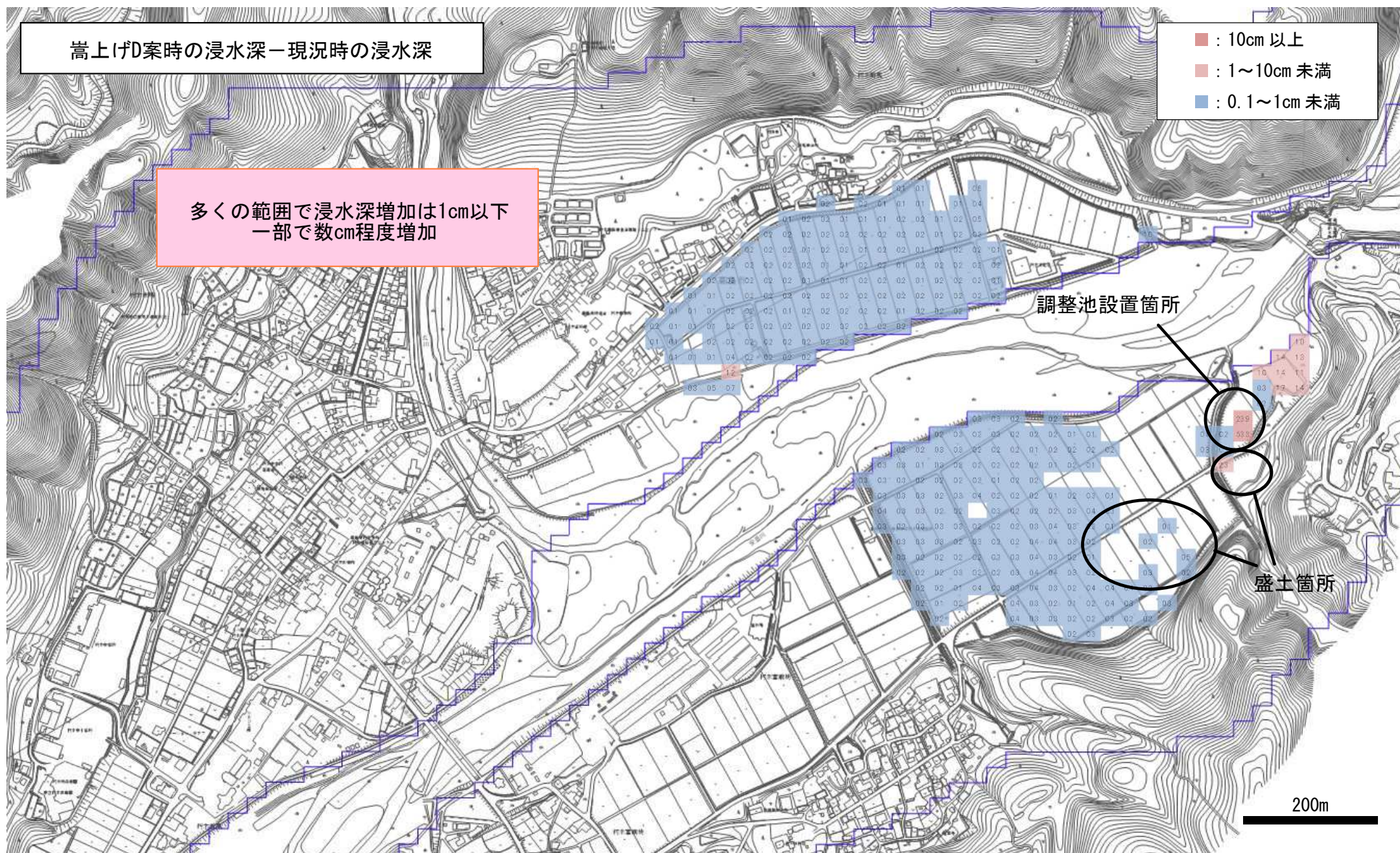
嵩上げD案時と現況時の浸水深差分図（平成25年9月流量）
