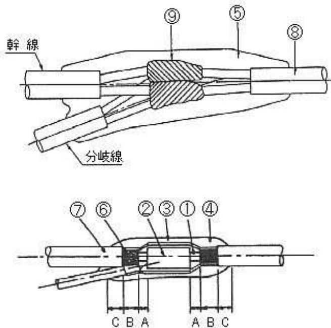
線心接続部
