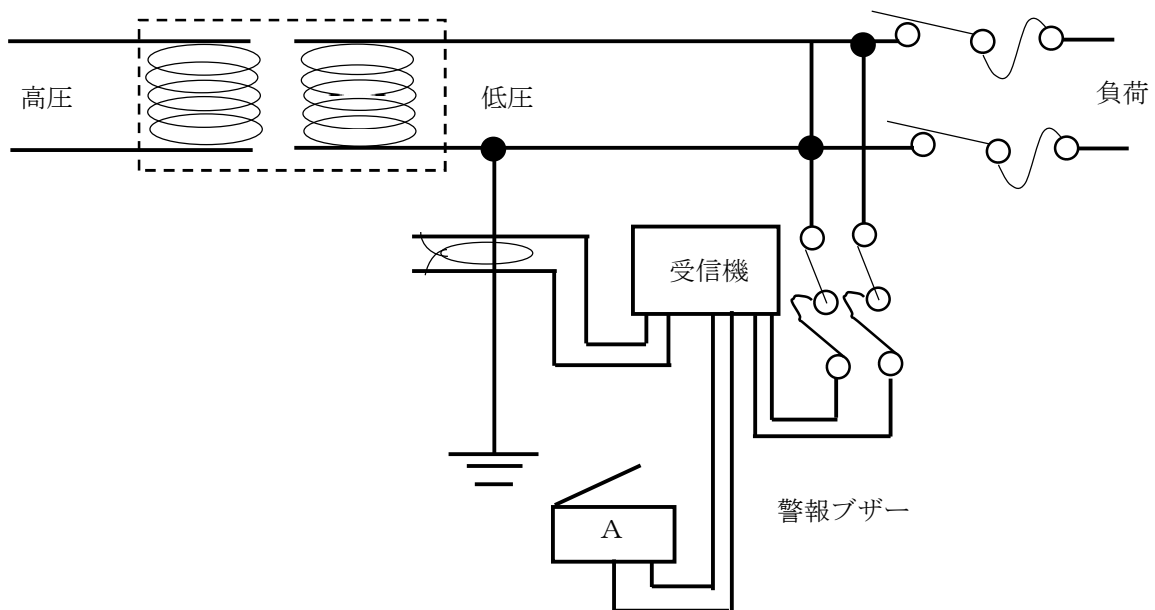
例 3 変圧器の B 種接地線に設ける方式の設置例 単相変圧器の B 種接地線に設ける場合 第 2 6 - 5 図
