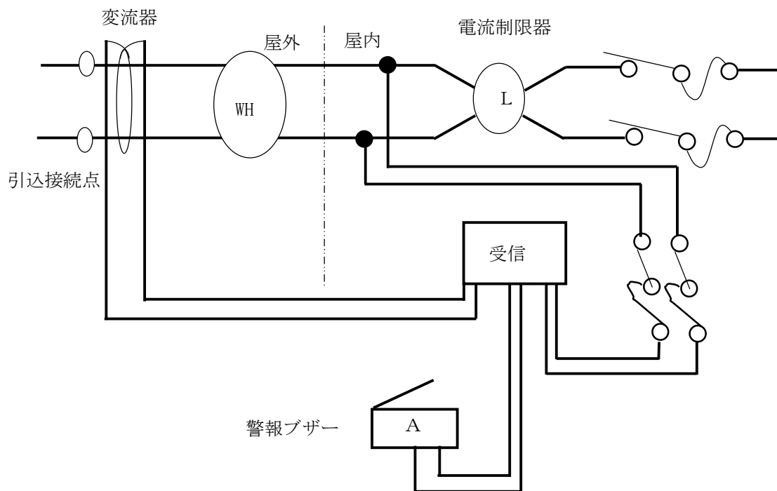
例 2 低圧による引込方式の設置例 変流器を屋外に設けた場合 第 2 6 - 3 図
