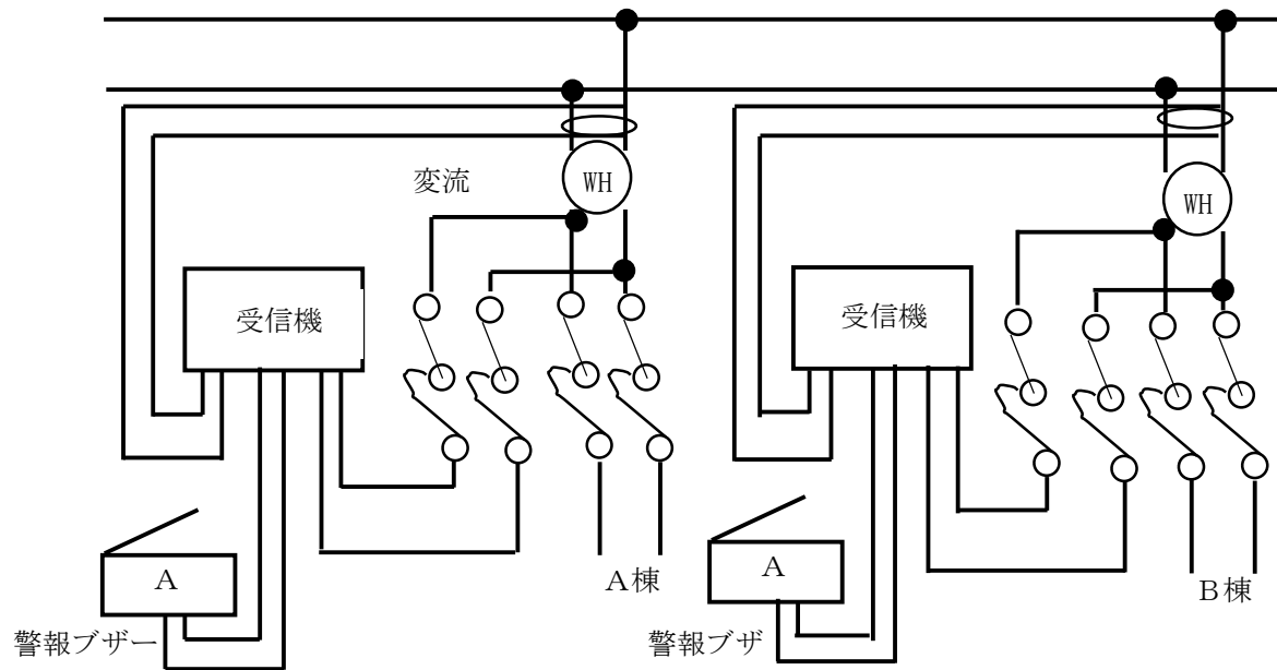
接続引込線が電気事業者の財産である場合 第 2 6 - 2 図
