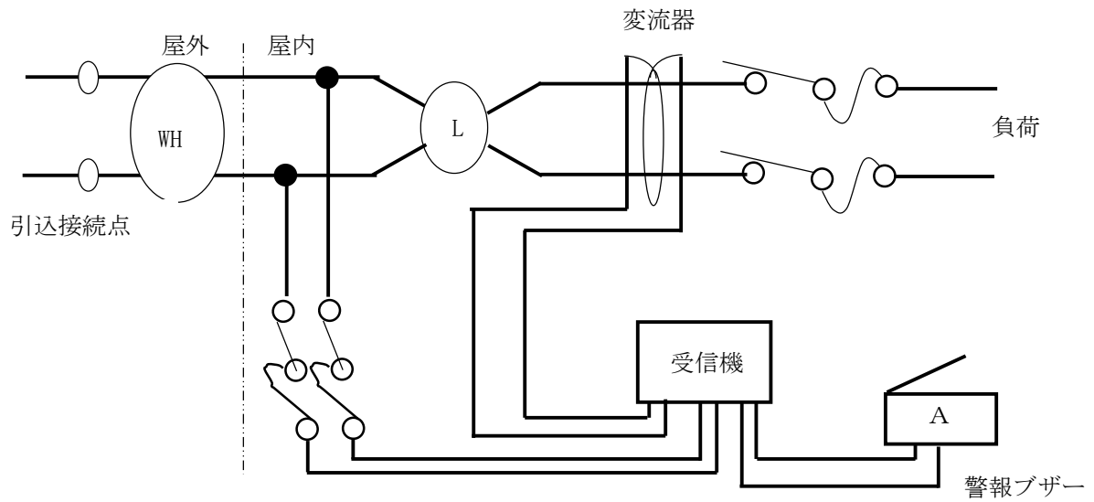
変流器を屋内に設けた例 第 2 6 - 4 図
