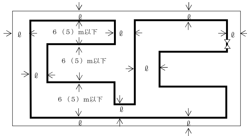
第 2.4-6.7 図 一辺省略と二辺省略の組合せの例 1
