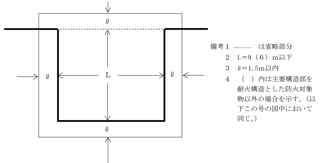
第 2 4 - 6 3 図 一辺省略の例 1
