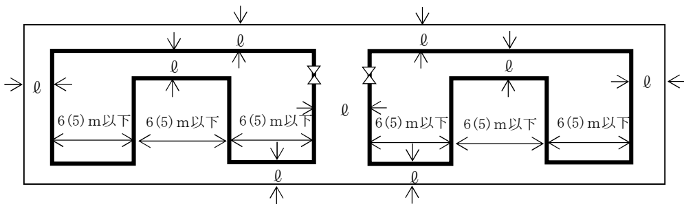
第 2.4-6.8 図 一辺省略と二辺省略の組合せの例 2（特に広い居室の場合）
