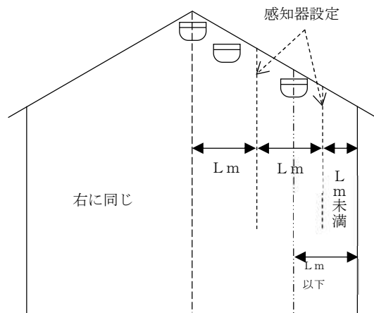
第 2 4 - 3 8 図 (断面図)
