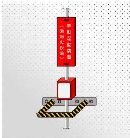
第 1 7 - 6 図 防護措置の例
